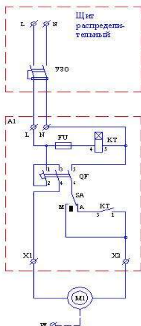
Эл.схема 1
